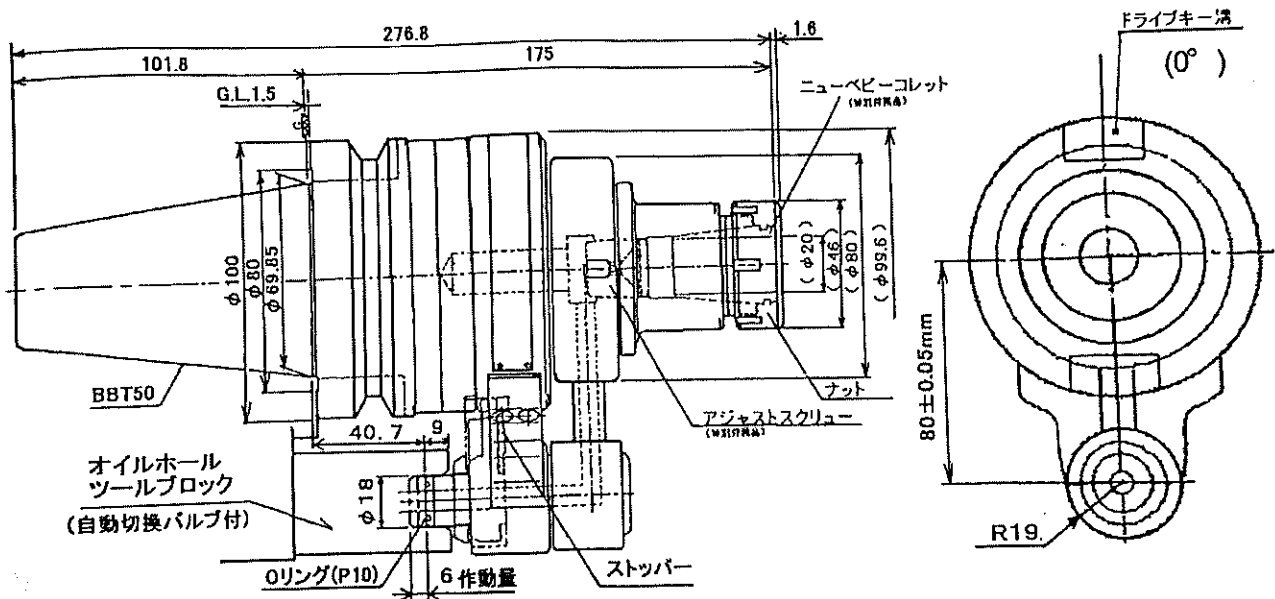
図1. ホルダ参考図 ( 図はB I G製:BT50-ONBS20N-175 の場合)
